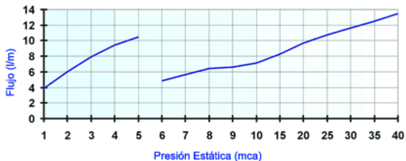
Curva de flujo x Presión de la Ducha
